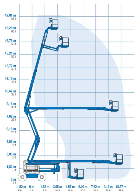
Arbeitsdiagramm Z-60/34
