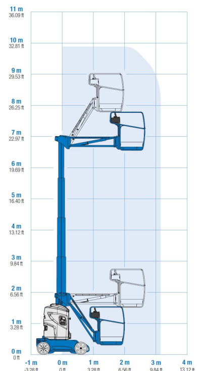
Arbeitsdiagramm GR-26J
